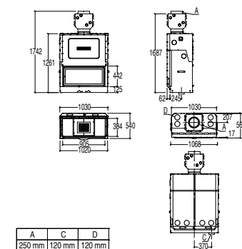
MA 263 SL PLUS
