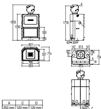
MA 261 SL PLUS CON MANTELLO CAPP (da montare in fase di installazione)
