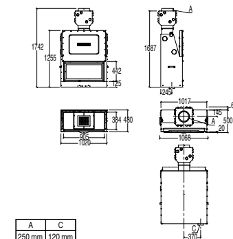
MA 263 SL PLUS CON MANTELLO CAPPA (da montare in fase di installazione)
