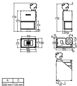
MA 283 D/S SL PLUS
