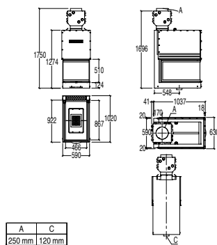
MA 272 SL PLUS
