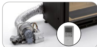
Kit di ventilazione Multifuoco System Plus singolo o doppio con telecomando LCD
