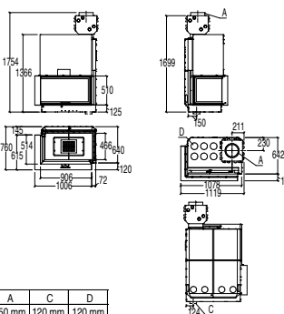
ME 90 D/S CON MANTELLO CAPPA (da montare in fase di installazione)
