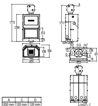
MA 260 SL PLUS CON MANTELLO CAPP (da montare in fase di installazione)
