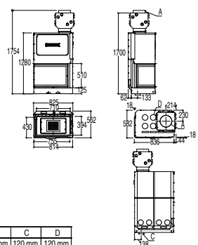
MA 285 D/S SL PLUS CON MANTELLO CAPPA (da montare in fase di installazione)
