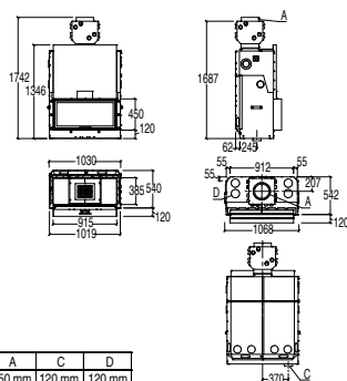
ME 90 B CON MANTELLO CAPPA (da montare in fase di installazione)
