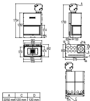
MA 283 D/S SL PLUS CON MANTELLO CAPP (da montare in fase di installazione)
