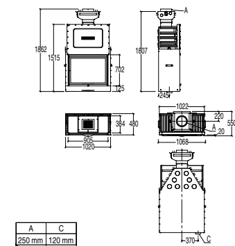
MA 262 SL PLUS
