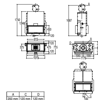
ME 90 CON MANTELLO CAPPA (da montare in fase di installazione)
