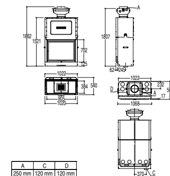
MA 262 SL PLUS CON MANTELLO CAPPA (da montare in fase di installazione)
