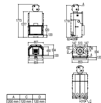
ME 70 CON MANTELLO CAPPA (da montare in fase di installazione)
