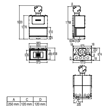
MA 271 SL PLUS CON MANTELLO CAPP (da montare in fase di installazione)
