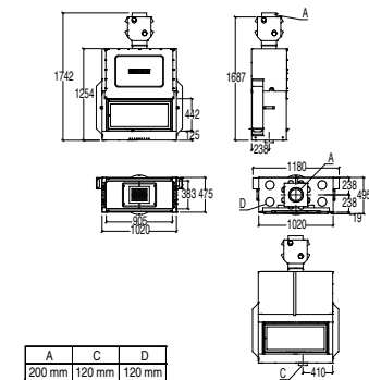
MA 263 B SL PLUS CON MANTELLO CAPP (da montare in fase di installazione)
