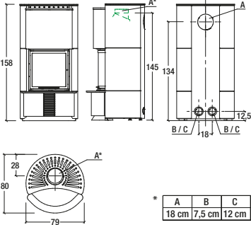
Model: C DUE
