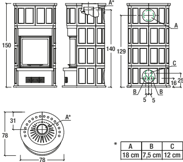
Model: C UNO
