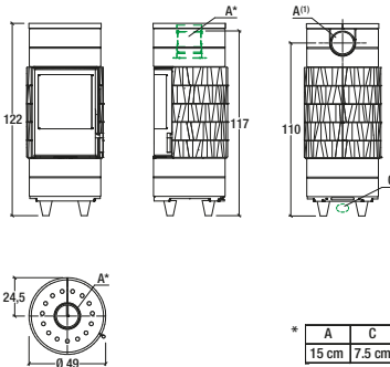
Model: CIRCLE BCS
