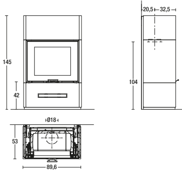
Model: BERN A
