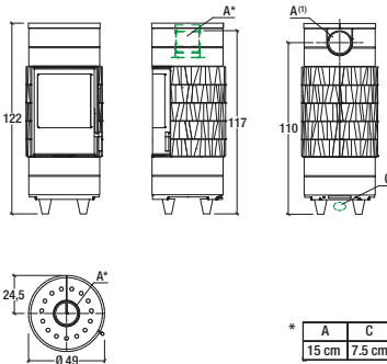
Model: CIRCLE Hermetic
