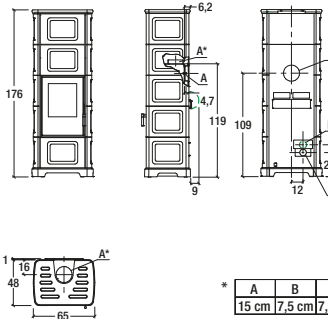
Model: E928 C-M BCS
