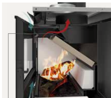
3- AVEC LA PORTE OUVERTE. Le clapet By-Pass est complètement ouvert et les fumées se dirigent rapidement vers le conduit de fumée.
