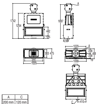
MA 263 B SL PLUS
