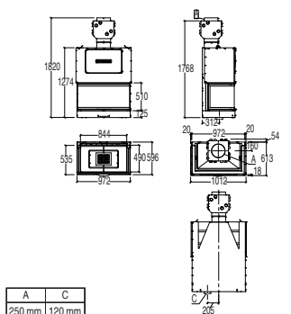
MA 271 SL PLUS
